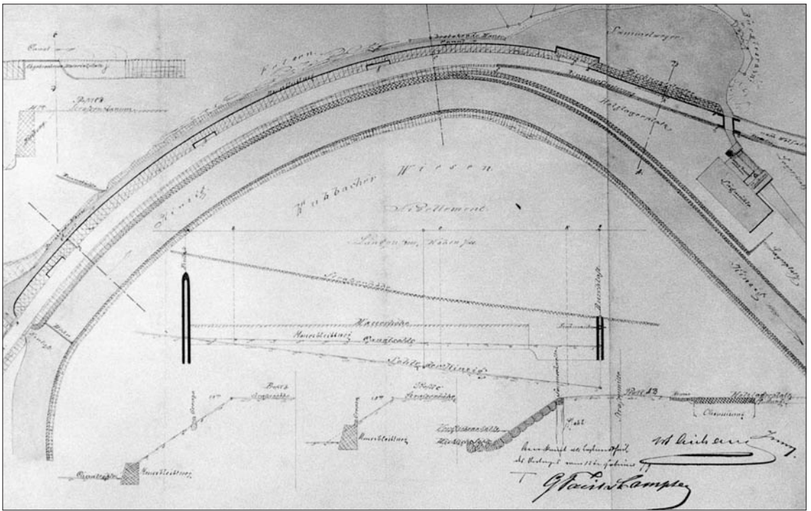
Abb. 1: Situationsplan des Sägewerks Faist & Compter in Schiltach mit Kanal und Sammelweiher vom 12. Februar 1879. Ganz links ist das Wehr in der Kinzig mit dem Einlass in den Kanal eingezeichnet. Kanal und Uferbogen des Sammelweihers (rechts oben) entsprechen dem Verlauf des alten Kinzigbetts. Die Gebäude der Säge befinden sich zwischen der Kinzig und der Straße nach Wolfach (rechts). Stadtarchiv Schiltach
